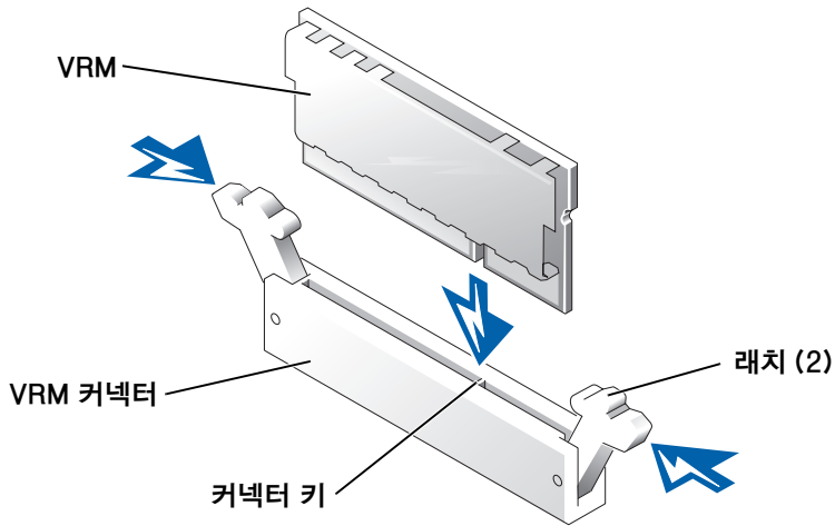
그림 6-2. VRM 설치
